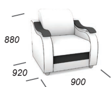
Габаритные размеры
