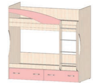
КРОВАТЬ 2х ЯРУСНАЯ 1892(Ш)х982(Г)х1855(В) мм размер под матрас 800х1860 мм универсальная сборка на любую сторону
