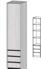
ПЕНАЛ 3 ЯЩИКА 500(Ш)х560(Г)х2200(В) мм
