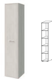
Пенал с полками ГШ-4 400x2160x500
